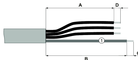
1 Προστατευτική γείωση (κίτρινο/πράσινο)
